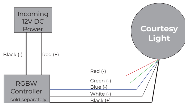
RGBW Wiring
